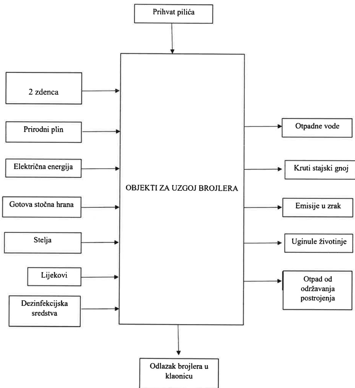
Prilog 2. Blok dijagram tehnološkog procesa novog postrojenja za intenzivan uzgoj peradi Farma Komarnica Ludbreška
